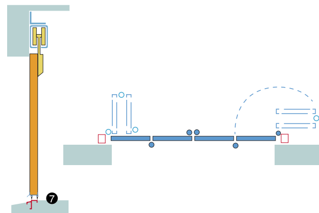
sistema anti-infiltrazione
