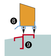
sistema anti-infiltrazione
